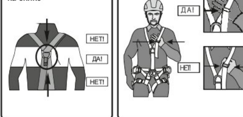
Рис. 10. Страховочная система
