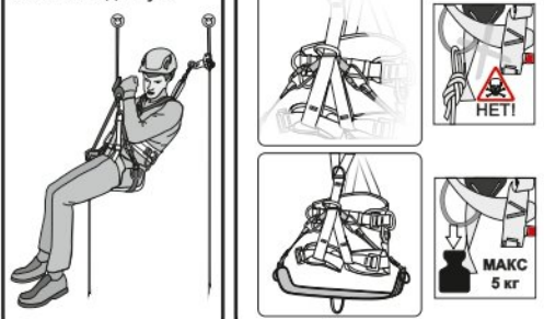
Рис. 13. Пример организации системы канатного доступа
